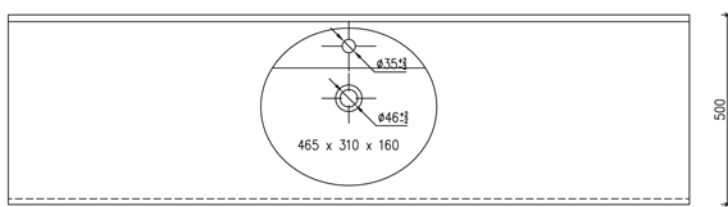
TOPLINE TREND 46/31 Art.Nr. 11570 Tiefe: ab 500 mm Becken: 465 x 310 x 160H mm Spritzkante / Frontschürze variabel
