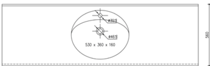
TOPLINE COMFORT 53/36 Art.Nr. 11550 Tiefe: ab 560 mm Becken: 530 x 360 x 160H mm Spritzkante / Frontschürze variabel
