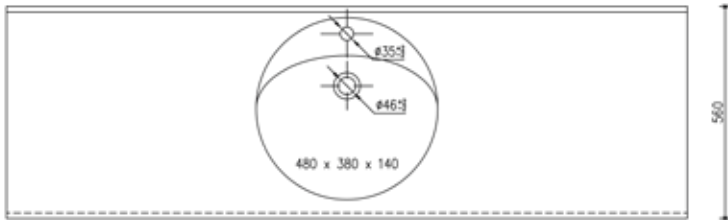
TOPLINE DISKUS 48 Art.Nr. 11620 Tiefe: ab 530 mm Becken: 480 x 380 x 140H mm Spritzkante / Frontschürze variabel
