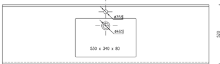
TOPLINE ELEMENT 53/34 Art.Nr. 11812 Tiefe bei axialer Armatur: ab 520 mm Tiefe bei seitlicher / Wandarmatur: ab 450 mm Becken: 530 x 345 x 80H mm Spritzkante / Frontschürze variabel
