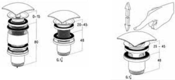
2a) Quadro Art.Nr. 20050 (feststehend ohne Überlaufbohrung im Becken) 2b) Quadro PopUp Art. Nr. 20055
