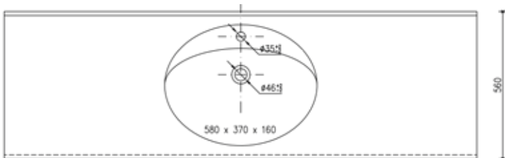
TOPLINE COMFORT 58/37 Art.Nr. 11560 Tiefe: ab 560 mm Becken: 580 x 370 x 160H mm Spritzkante / Frontschürze variabel
