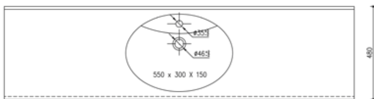
TOPLINE ACCESS Art.Nr. 11650 Tiefe: ab 480 mm Becken: 550 x 300 x 150H mm Spritzkante / Frontschürze variabel
