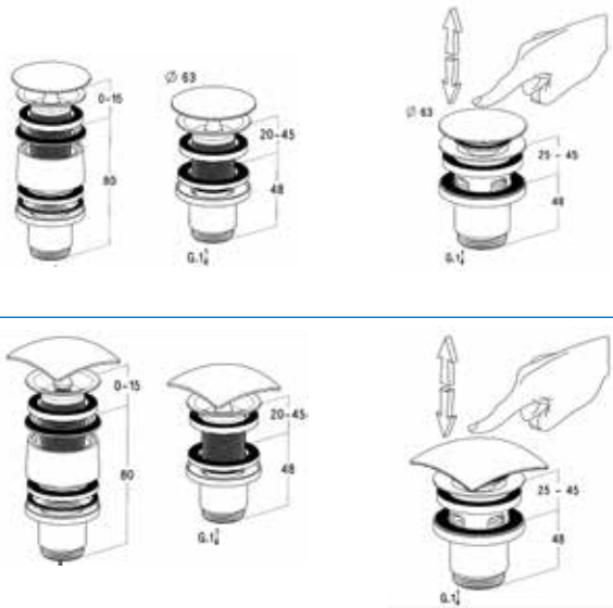
Design Ablauf verchromt, mit rundem Deckel 1a)Rondo Art Nr. 20035 (feststehend ohne Überlaufbohrung im Becken) 1b) Rondo PopUp Art Nr. 20040 1c)Rondo für Excenter Art Nr. 20045
