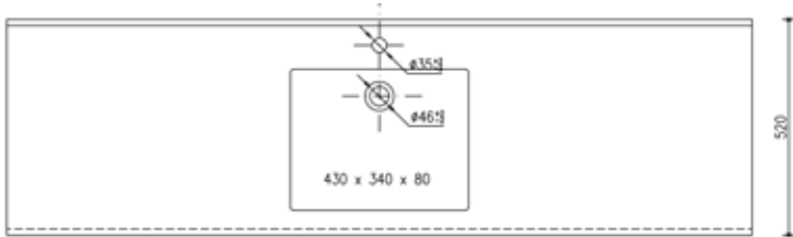
TOPLINE ELEMENT 43/34 Art.Nr. 11810 Tiefe bei axialer Armatur: ab 510 mm Tiefe bei seitlicher / Wandarmatur: ab 440 mm Becken: 430 x 340 x 80H mm Spritzkante / Frontschürze variabel
