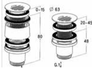
Design Siebablauf Art.Nr. 20030
