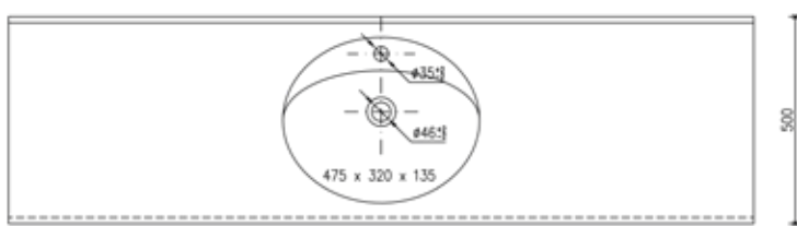
TOPLINE COMFORT 47/32 Art.Nr. 11545 Tiefe: ab 500 mm Becken: 475 x 320 x 135H mm Spritzkante / Frontschürze variabel
