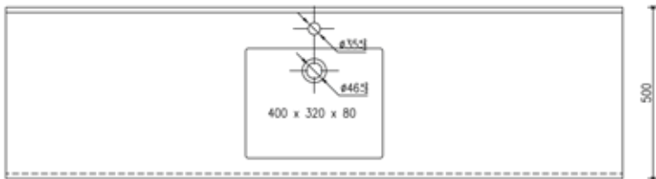
TOPLINE ELEMENT 40/32 Art.Nr. 11808 Tiefe bei axialer Armatur: ab 490 mm Tiefe bei seitlicher / Wandarmatur: ab 420 mm Becken: 400 x 320 x 80H mm Spritzkante / Frontschürze variabel
