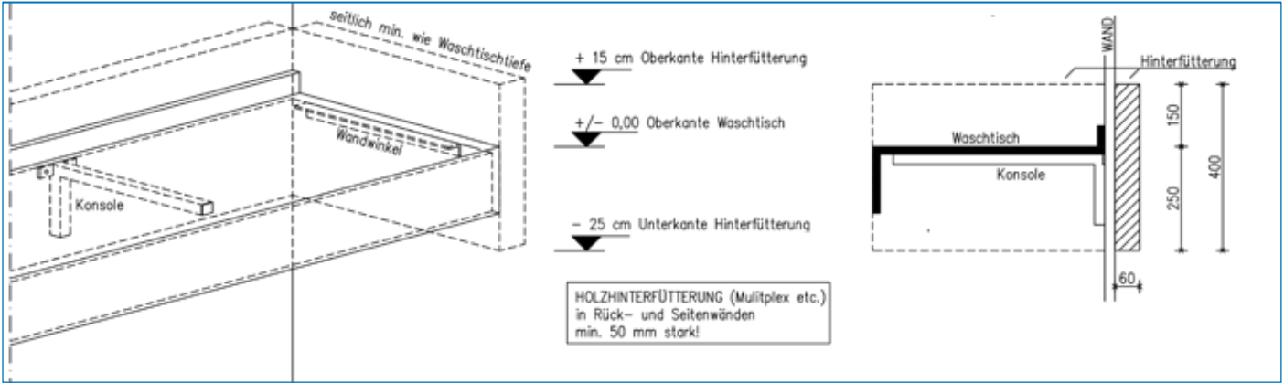
VIERKANT-KONSOLE 25 mm Art.Nr. 21000 Bohrungen 9 mm pulverbeschichtet, weiß
