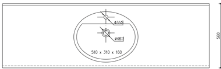
TOPLINE TREND 51/31 Art.Nr. 11575 Tiefe: ab 530 mm Becken: 510 x 310 x 160H mm Spritzkante / Frontschürze variabel
