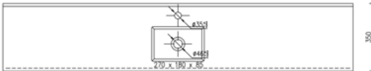
TOPLINE KUBIC 27/18 Art.Nr. 11335 Tiefe mit axialer Armatur: ab 350 mm Tiefe bei seitlicher / Wandarmatur: ab 280 mm Becken: 270 x 180 x 85H mm Spritzkante / Frontschürze variabel
