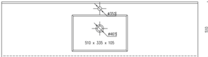
TOPLINE KUBIC 51/33 Art.Nr. 11338 Tiefe bei axialer Armatur: ab 510 mm Tiefe bei Wandarmatur: ab 440 mm Becken: 510 x 335 x 105H mm Spritzkante / Frontschürze variabel
